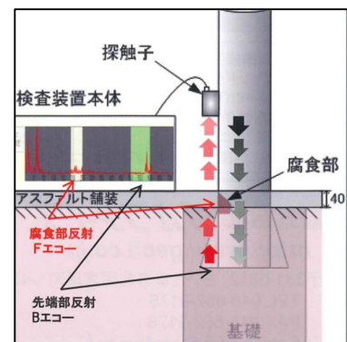
非破壊試験
