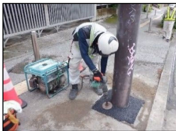
掘削点検状況（復旧材転圧）
