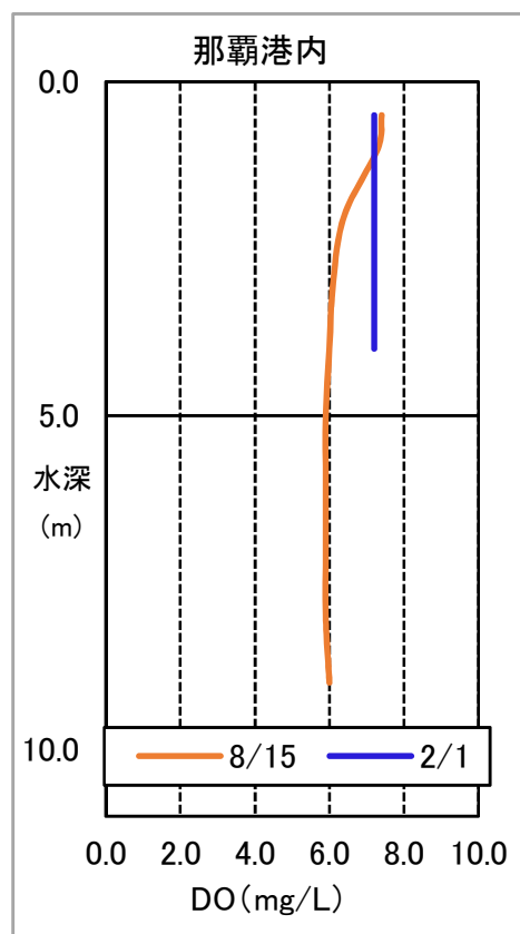
図 3-1 DO 鉛直分布
