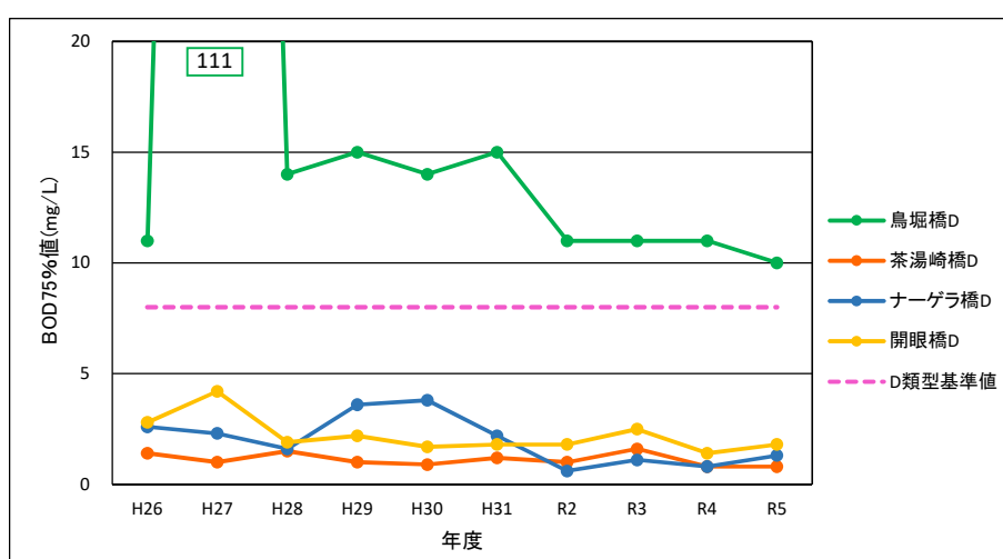
図 4-6 安里川の水質 (BOD75%値) 経年変化
