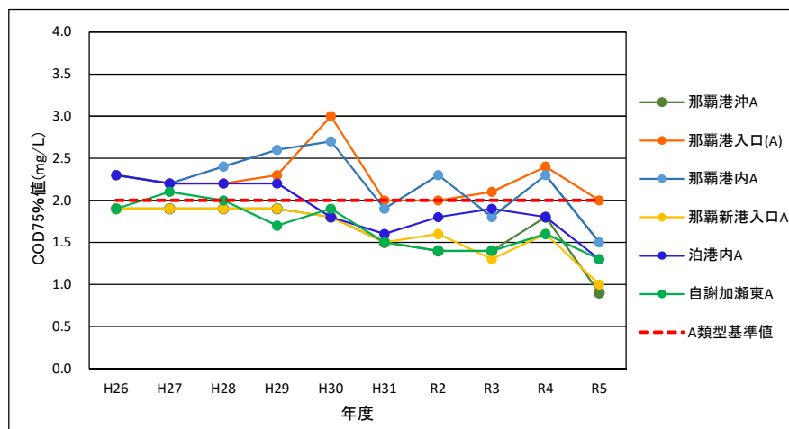
図 4-10 那覇港海域の水質 (COD75%値) 経年変化
