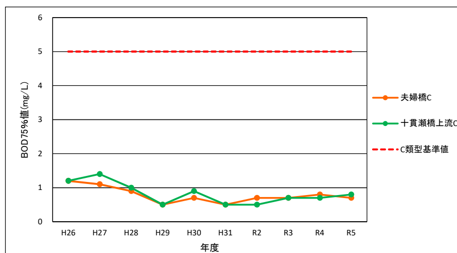
図 4-7 久茂地川の水質 (BOD75%値) 経年変化
