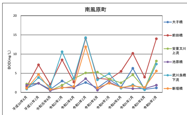
図 6-5 南風原町 BOD 経年変化
