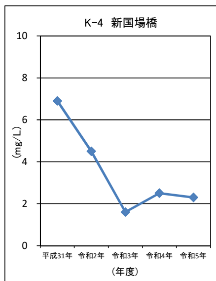
図 6-2 水質経年変化図 (BOD)
