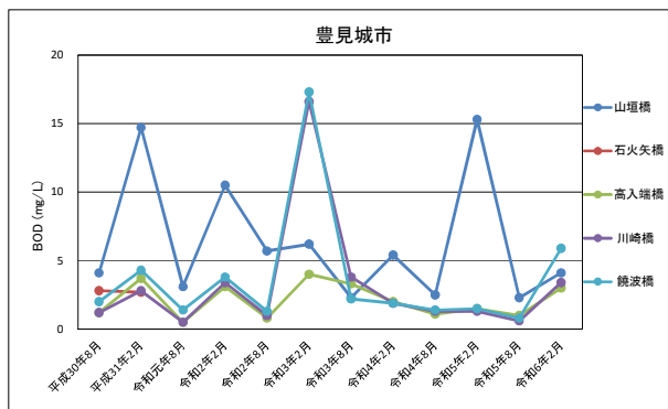
図 6-7 豊見城市 BOD 経年変化
