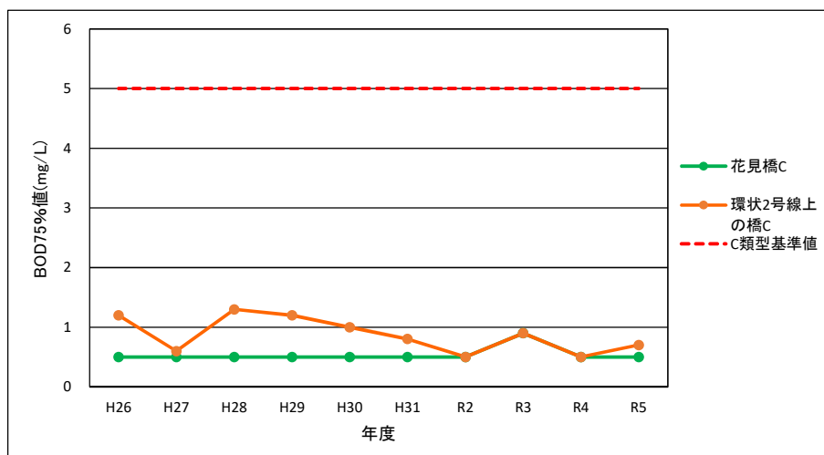
図 4-5 安謝川の水質 (BOD75%値) 経年変化
