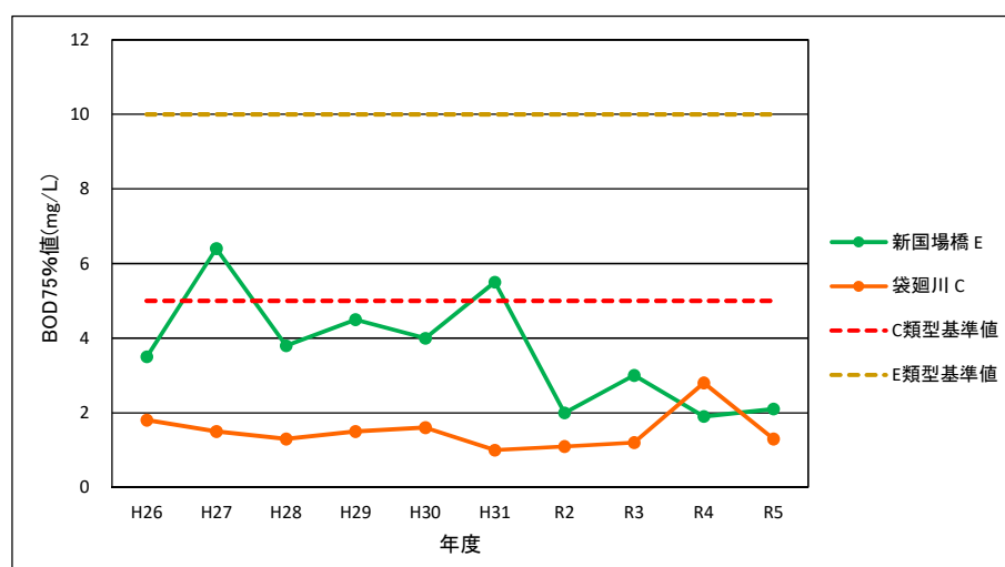
図 4-8 国場川の水質 (BOD75%値) 経年変化
