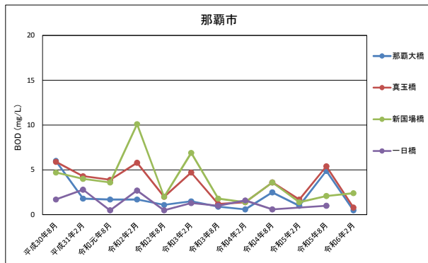
図 6-3 那覇市 BOD 経年変化
