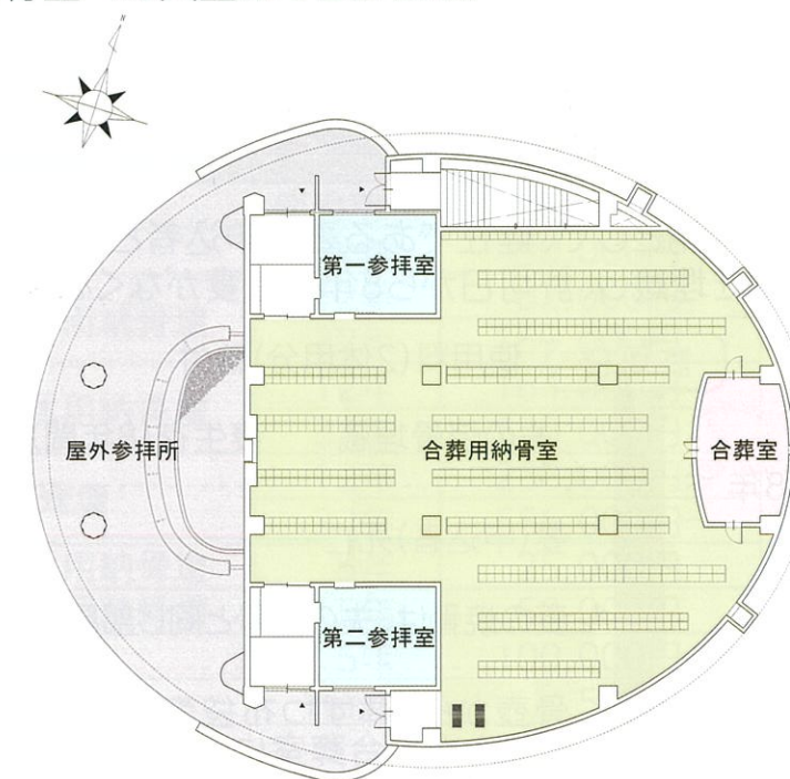
1階平面図
