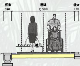
園路標準断面図
