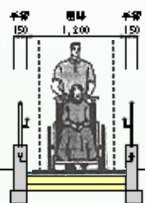
園路標準断面図
