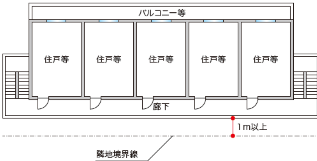
(廊下型特定共同住宅等(隣地境界線から廊下までの距離))
