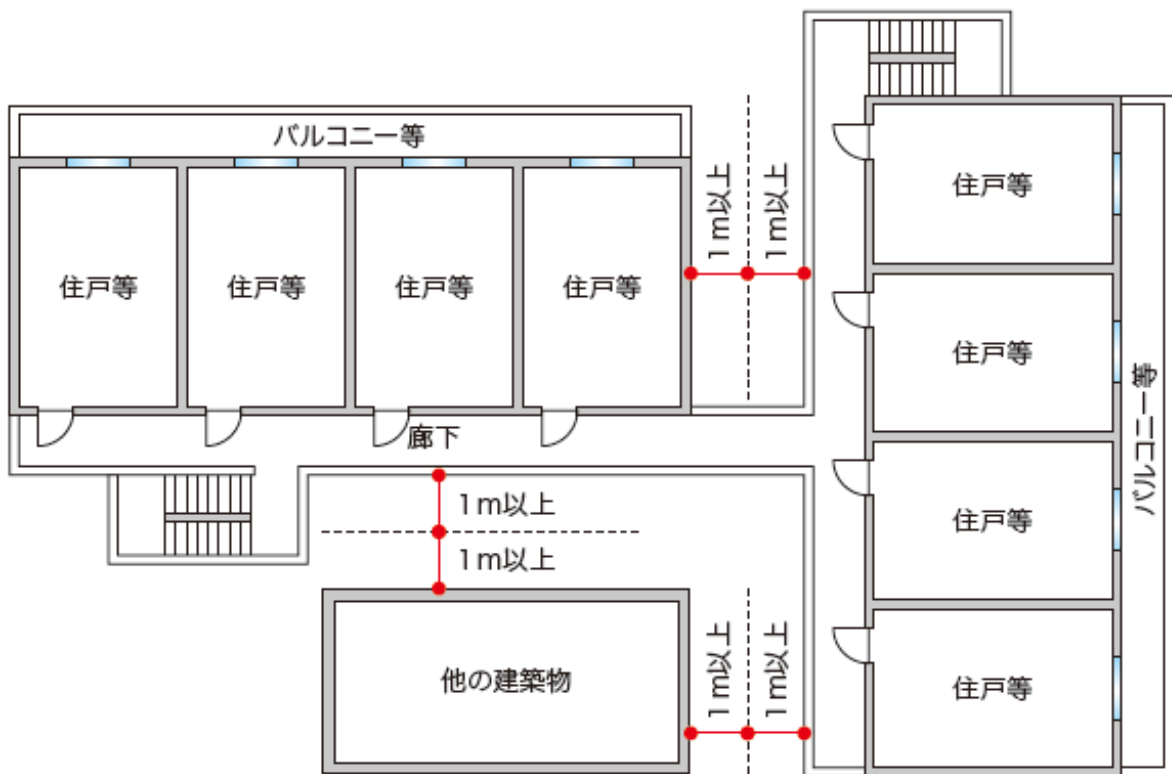
(廊下型特定共同住宅等(他の建築物等の外壁から廊下までの距離))
