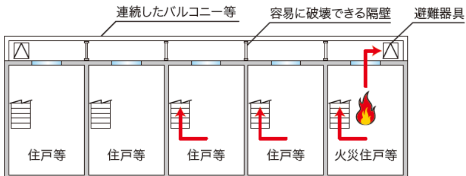
(メゾネット型住戸等の下階)
