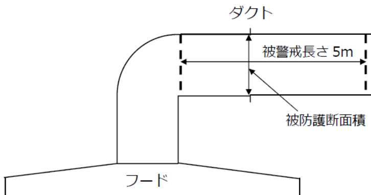
第 25-6 図 ダクトの被警戒長さ及び被防護断面積
