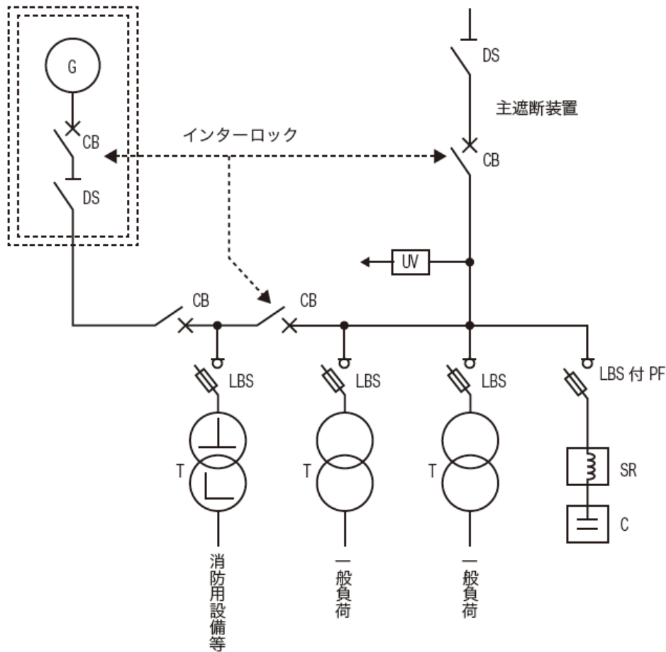
(高圧自家発電設備の例)
