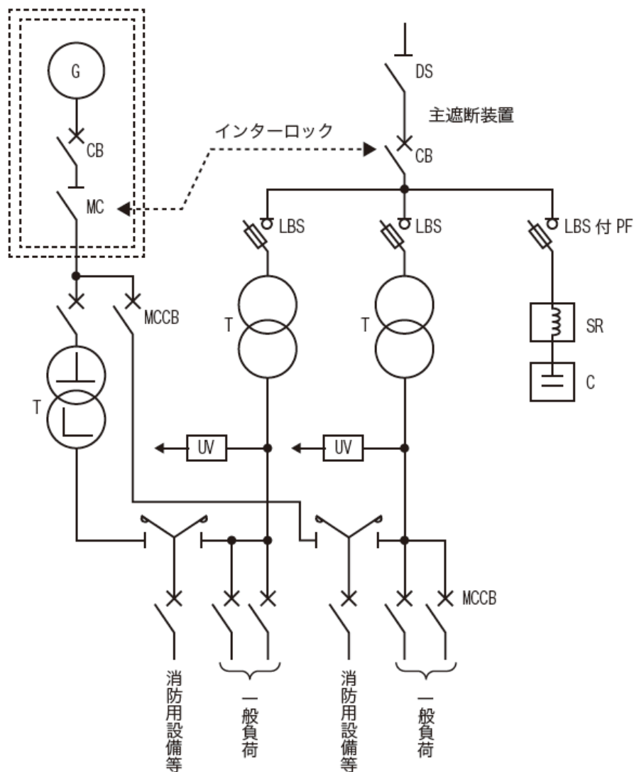
(低圧自家発電設備の例)
