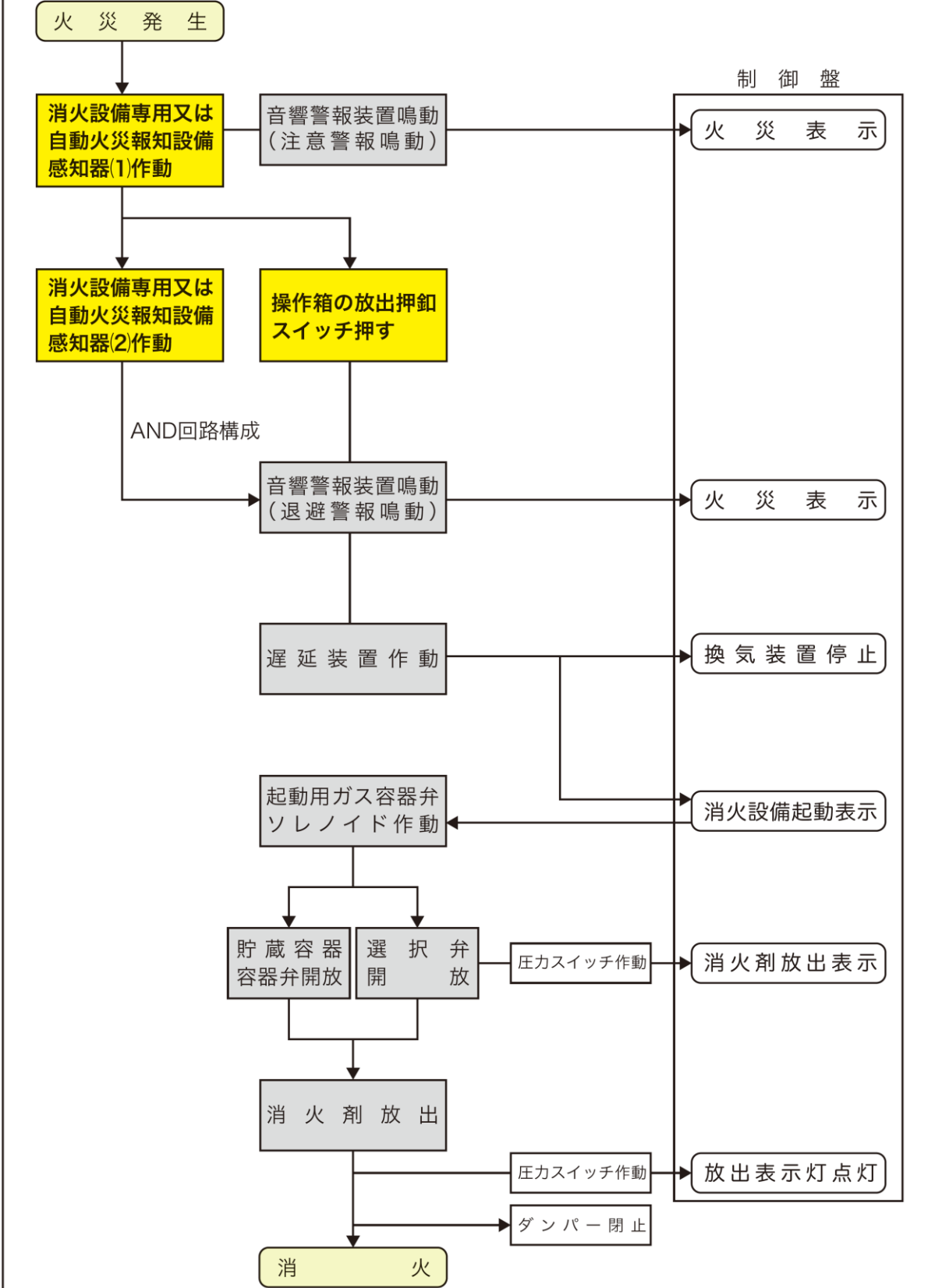
自動式の場合のフロー
