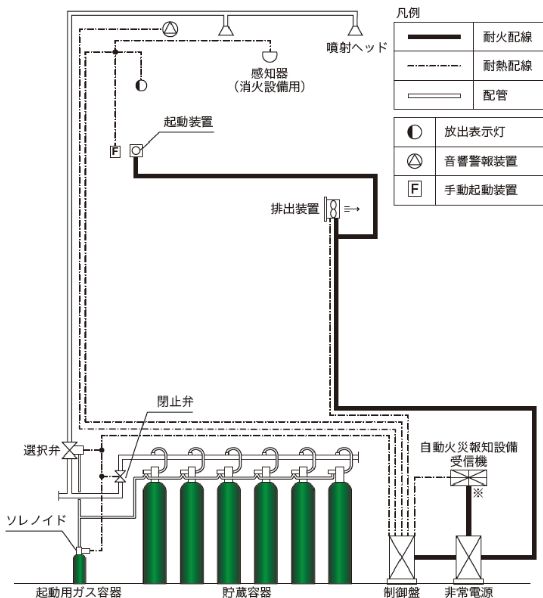
備考：蓄電池が内蔵されている場合、一次側配線（※）は、一般配線として差し支えない。 第5-22図
