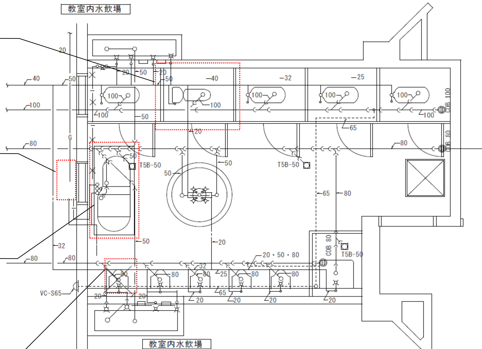
改修トイレ図面
