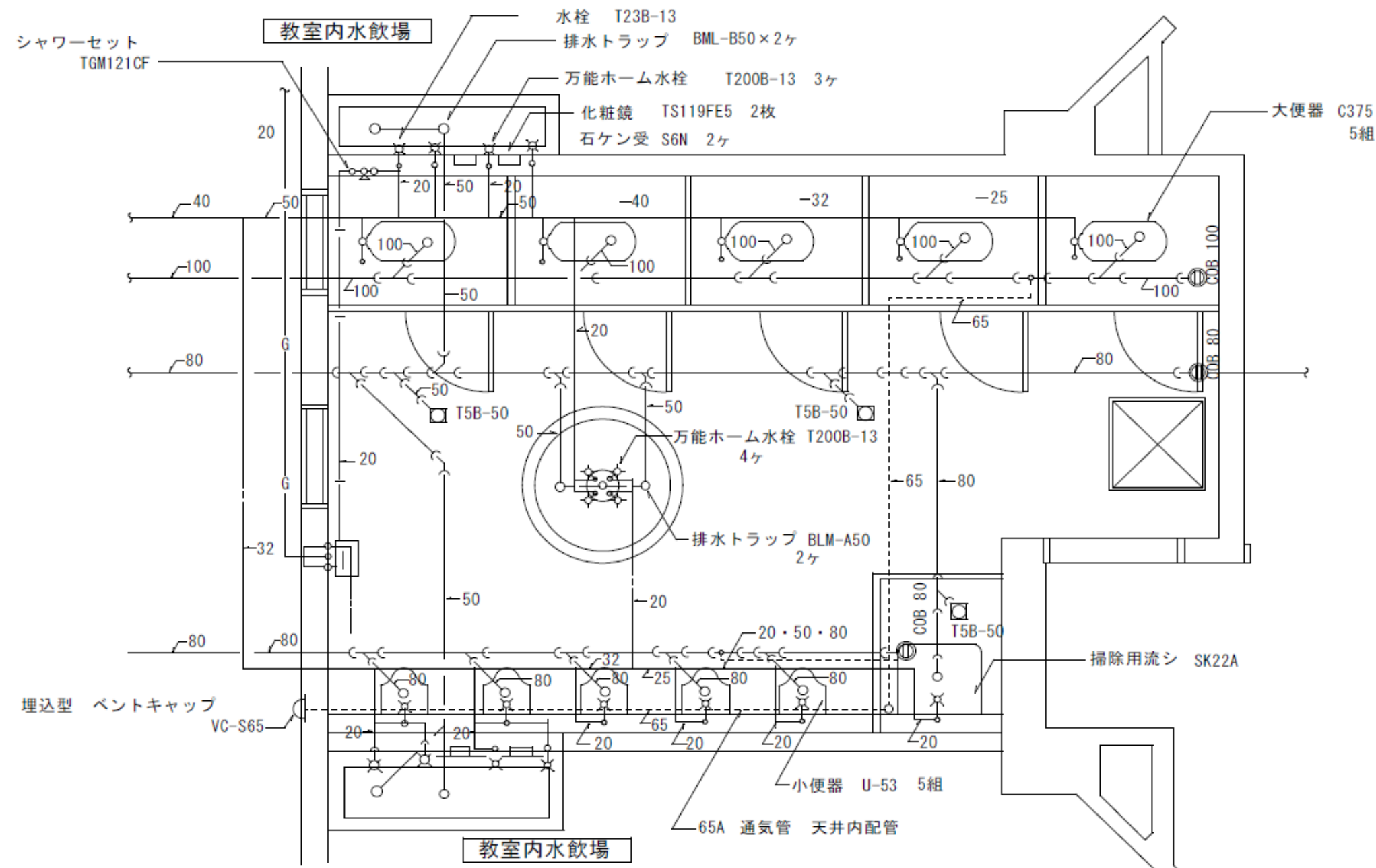
既設トイレ図面
