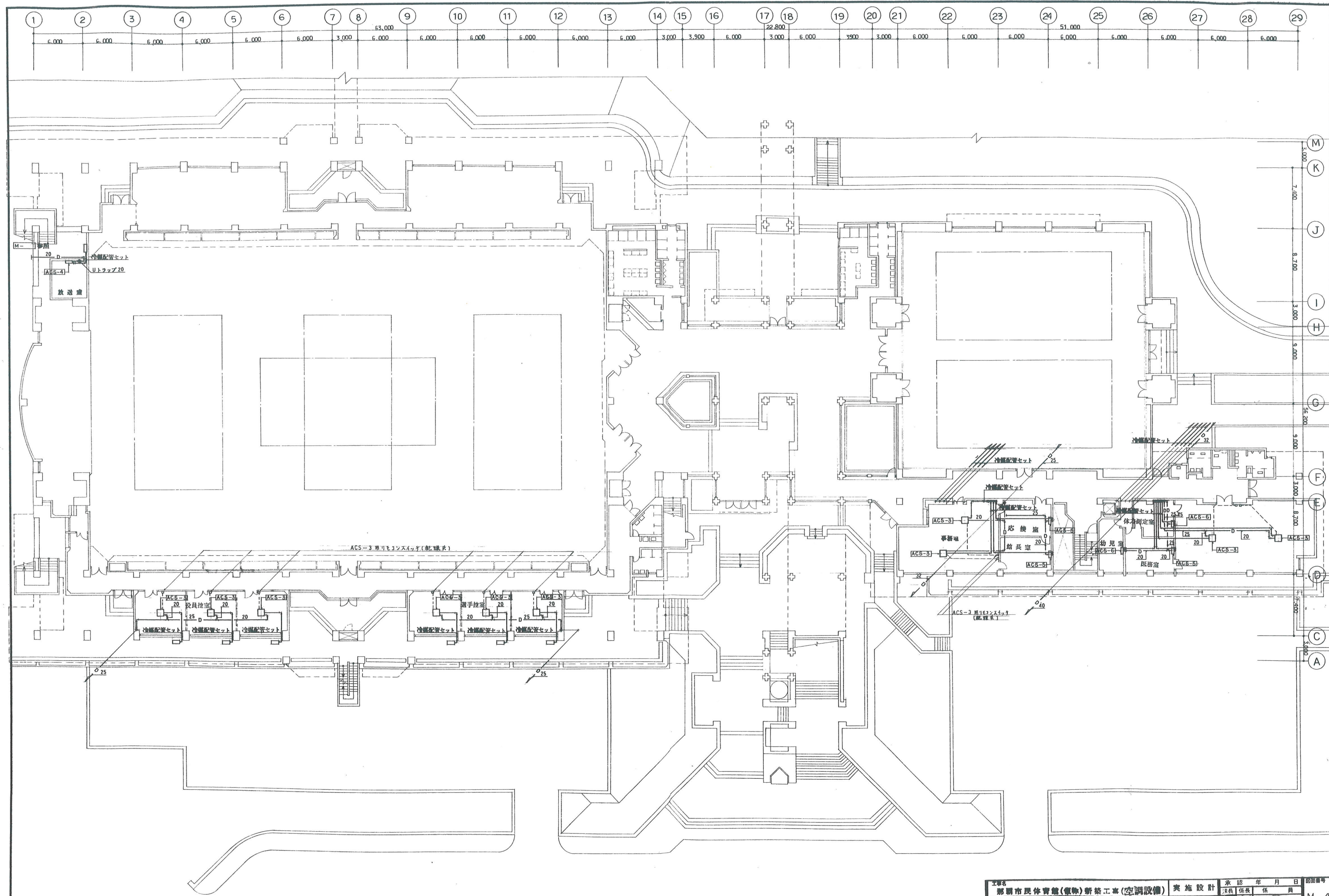
1階空調設備平面図 SCALE=1:200
