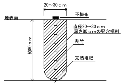
割竹挿入縦穴式土壌改良 断面図
