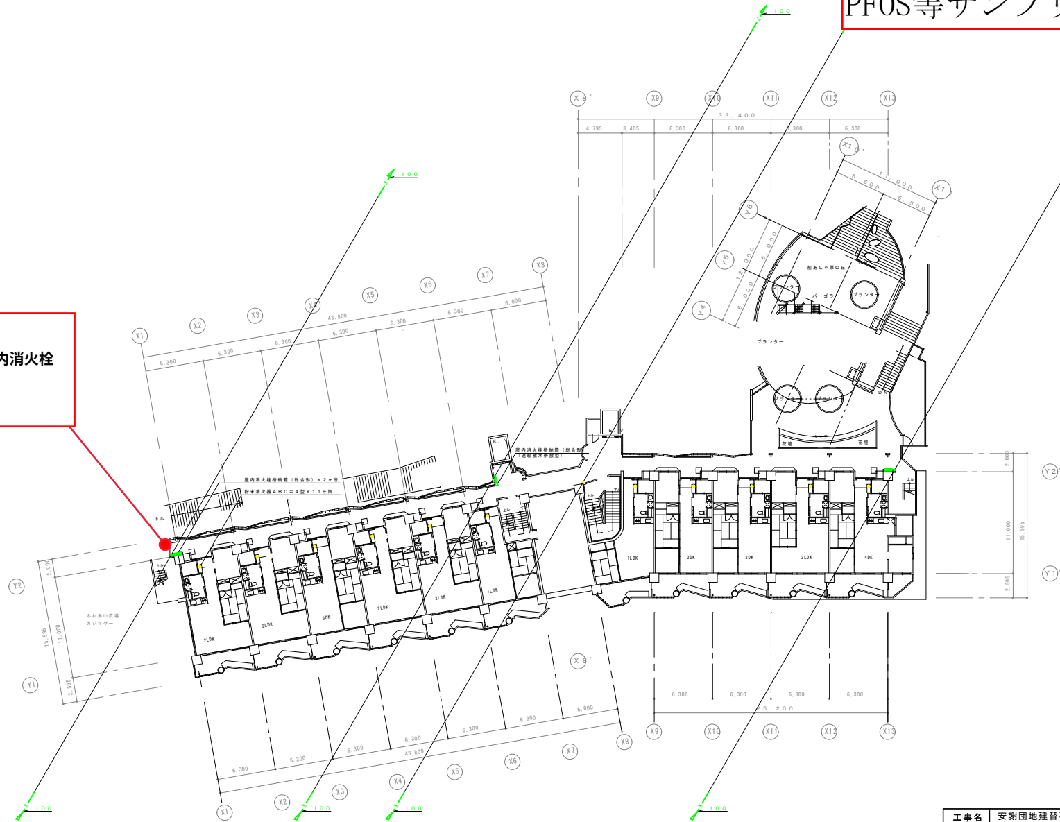
公営住宅高層棟3階平面図 S=1:200
