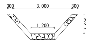
水路詳細図
