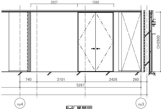
B-B' 展開図
