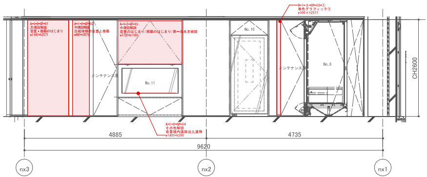
C-C' 展開図
