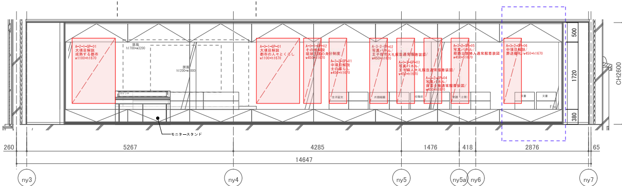
D-D' 展開図
