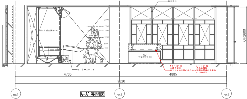
A-A' 展開図
