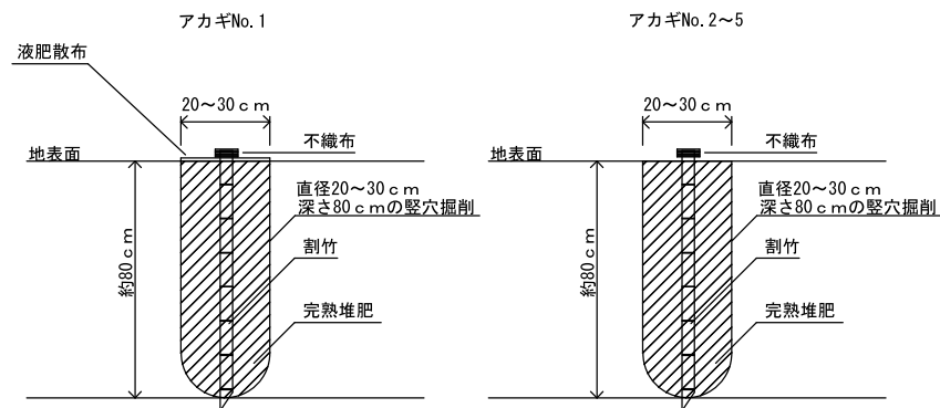
割竹挿入縦穴式土壌改良 断面図
