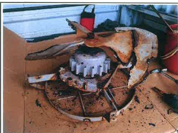
⑤既設ルーフファン腐食状況
