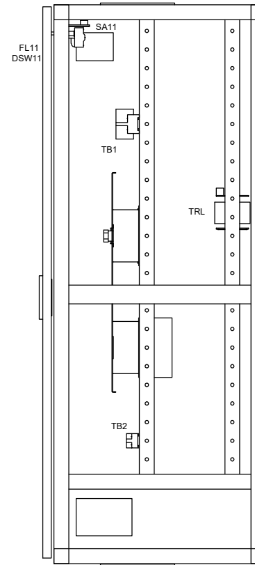
右側面
