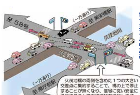
■久茂地橋交差点改良のポイント②
