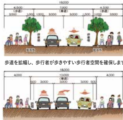
交差点改良を行うことで、交通混雑の緩和を図ります
