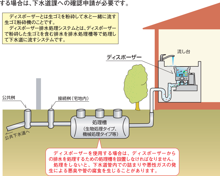
ディスポーザー排水処理システムのしくみ(生物処理タイプの例)
