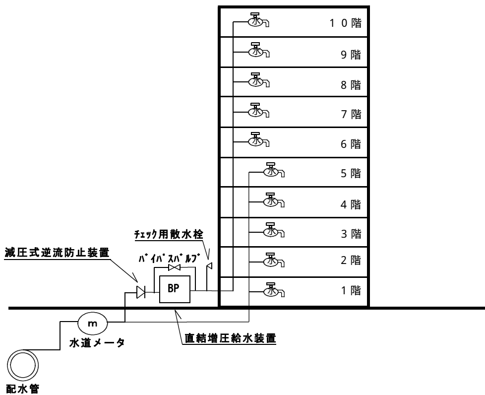
例 2．直結増圧給水装置での給水
