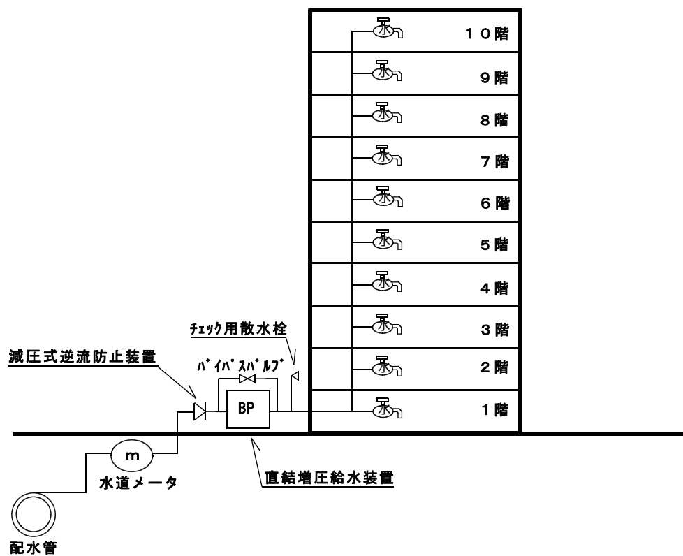
例 1．直結増圧給水装置での給水
