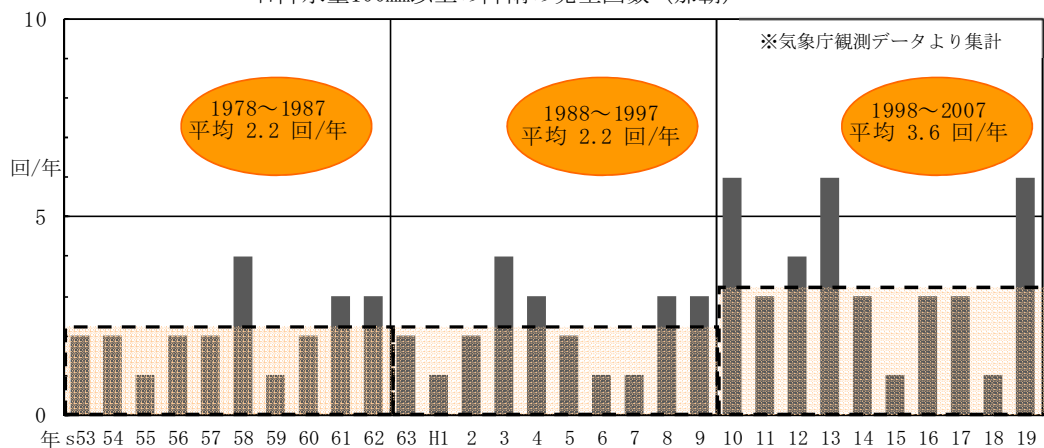
日降水量100mm以上の降雨の発生回数（那覇）
