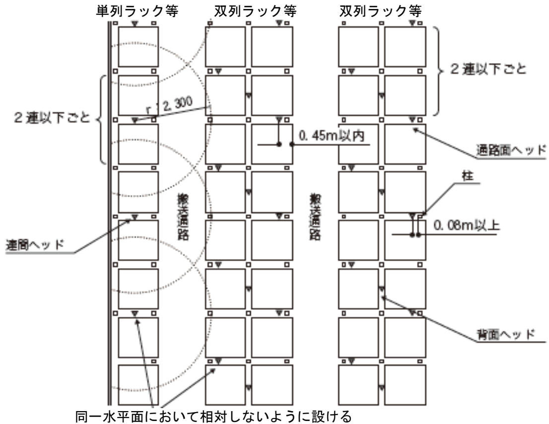
（平面図 レベル2、4 配置）
