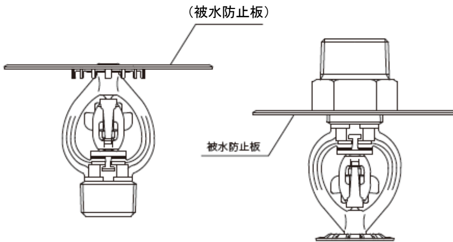
上向き型ヘッドの場合
