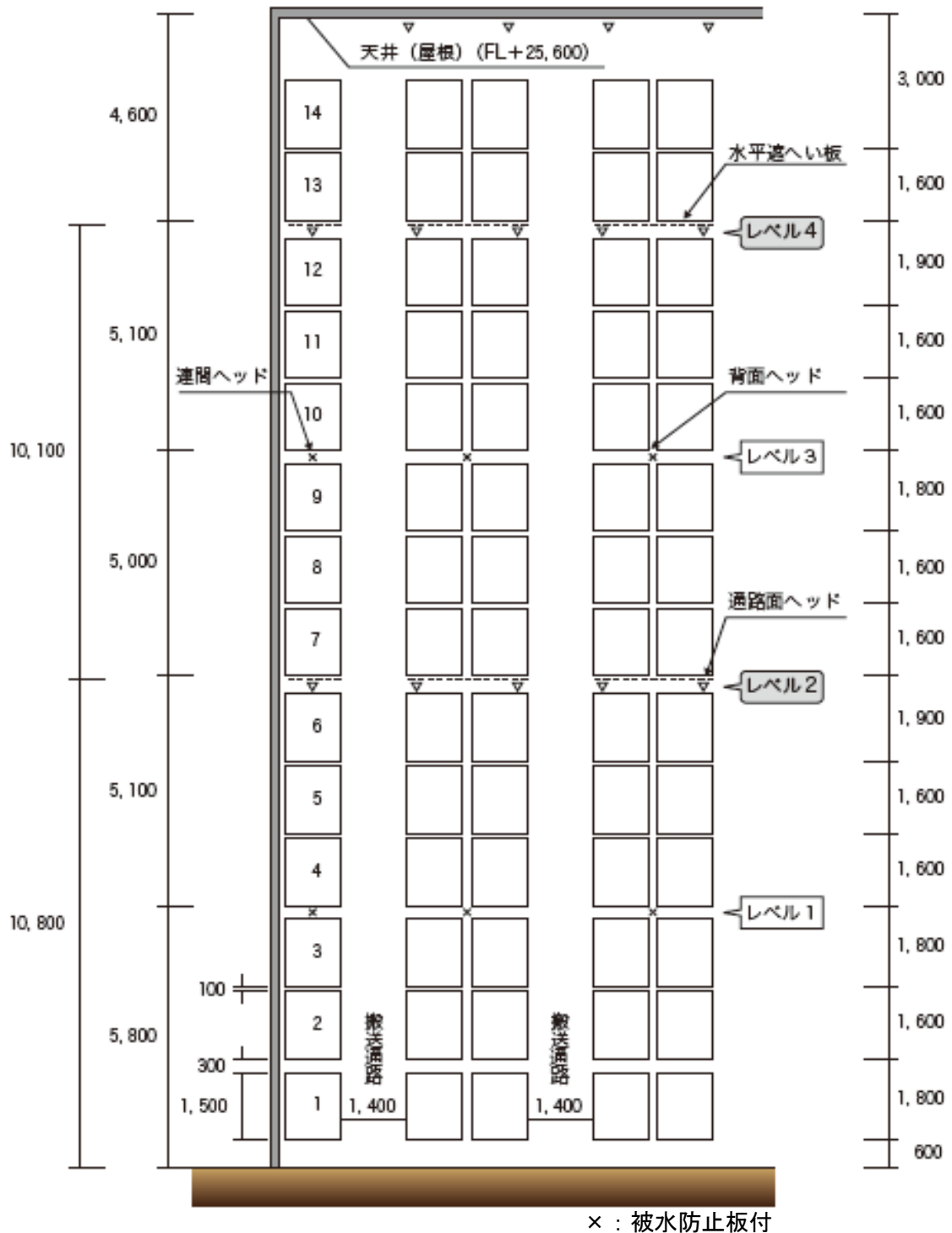
（断面図）
