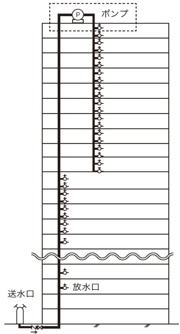
ポンプを屋上に設置したもの
