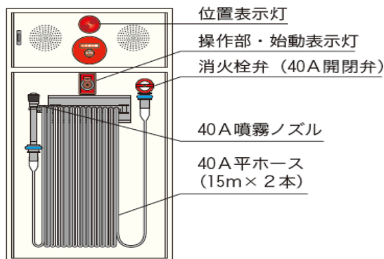
(1号消火栓(操作部から起動する方式)の構成例)
