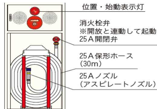
(広範囲型2号消火栓の構成例)
