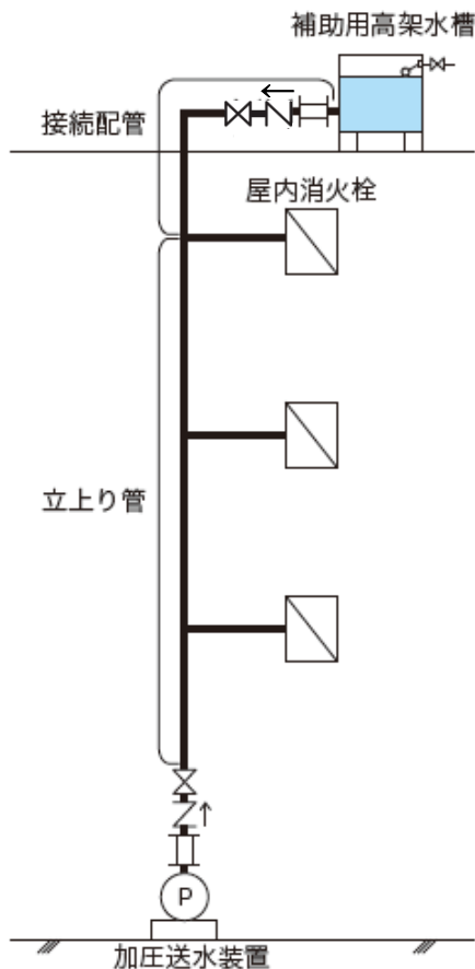
(補助用高架水槽による場合)
