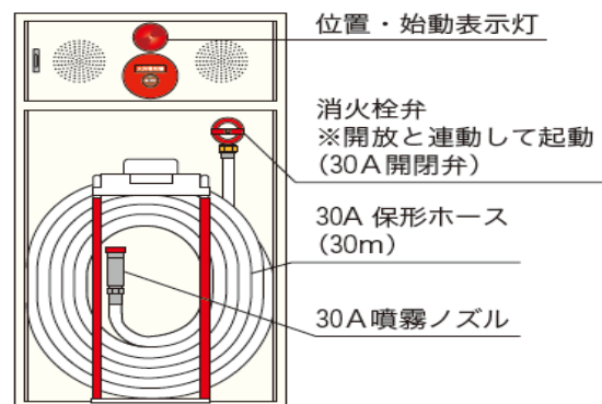
(易操作性1号消火栓の構成例)
