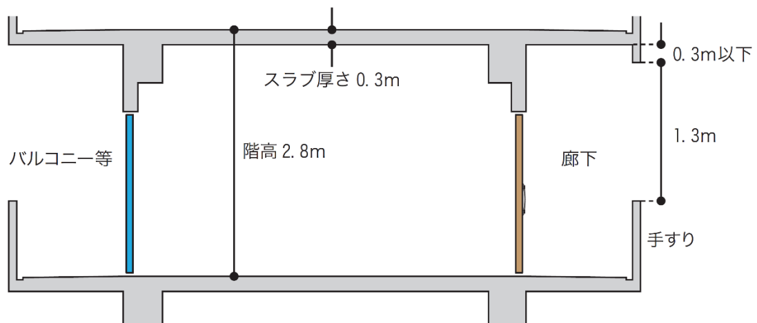
(断面図)
