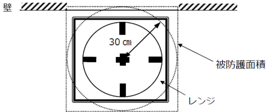
第 25-7 図 レンジの被防護面積（コンロが1口の場合）
