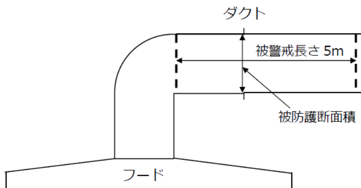
第 25－6 図 ダクトの被警戒長さ及び被防護断面面積
