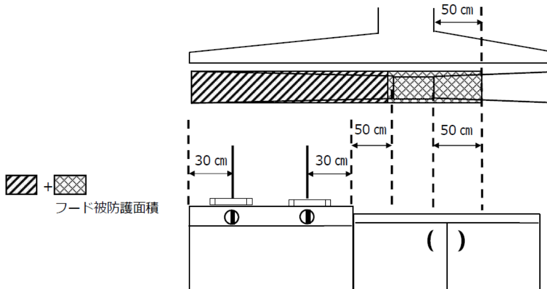
第 25－5 図 ダクト吸込口がレンジの直上部以外の位置にある場合のフードの被防護面積
