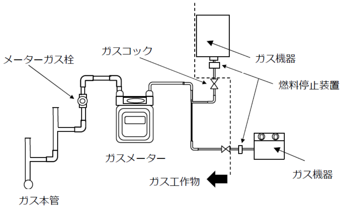
第 25－3 図 ガス燃料停止装置の設置位置（ガス事業者が設置する自動ガス遮断装置以外）
