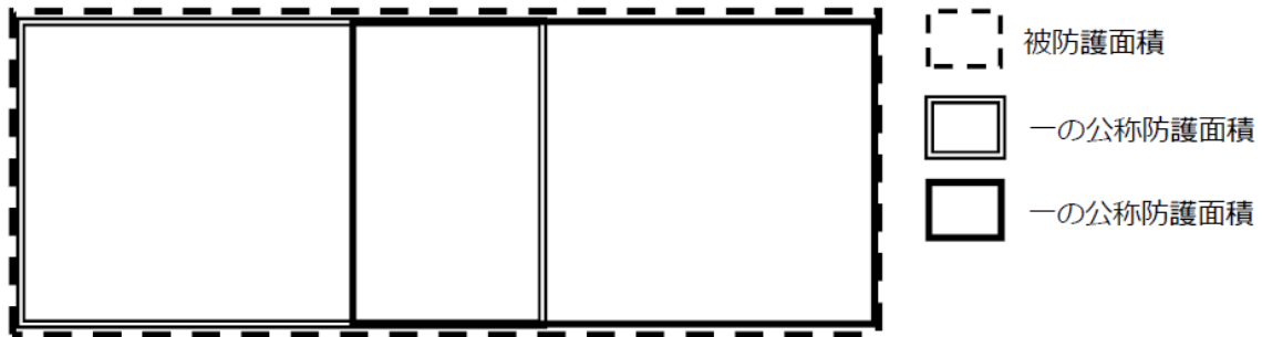
第 25-11 図 防護対象物が大きく一の装置で警戒できない場合
