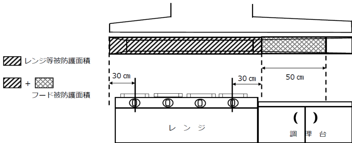
第 25－4 図 レンジ又はフライヤーの被防護面積よりフードが大きい場合のフードの被防護面積
