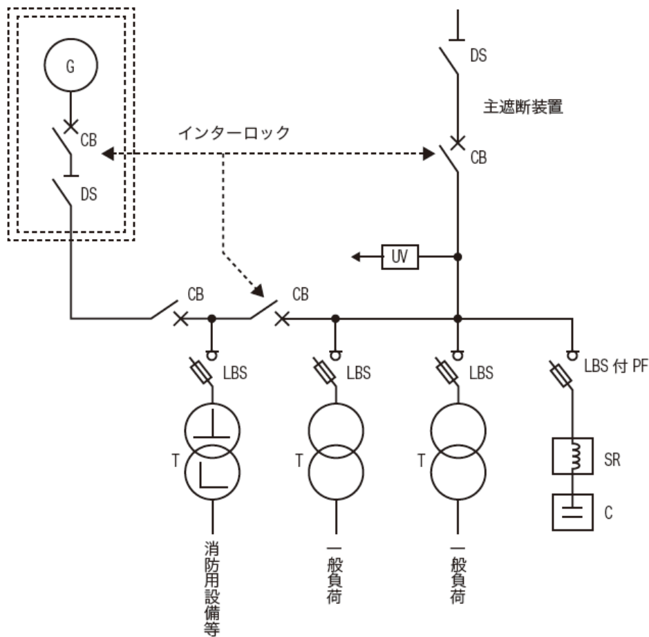
(高圧自家発電設備の例)
