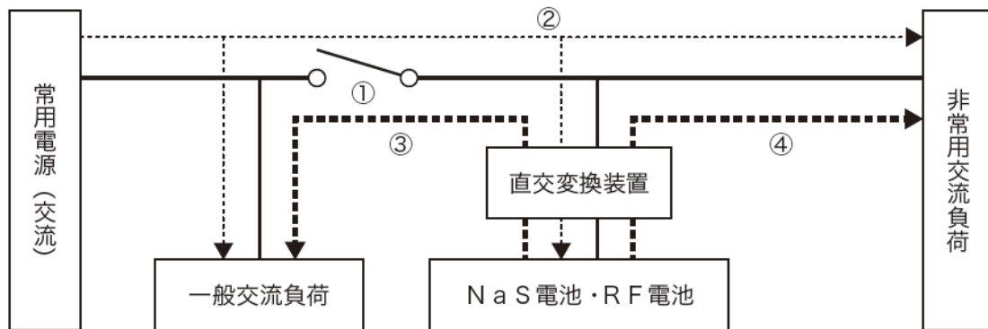
(直交変換装置の例)
