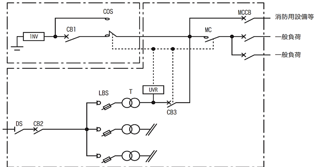
別図6 燃料電池設備（低圧発電設備で供給するもの）の分岐方法
