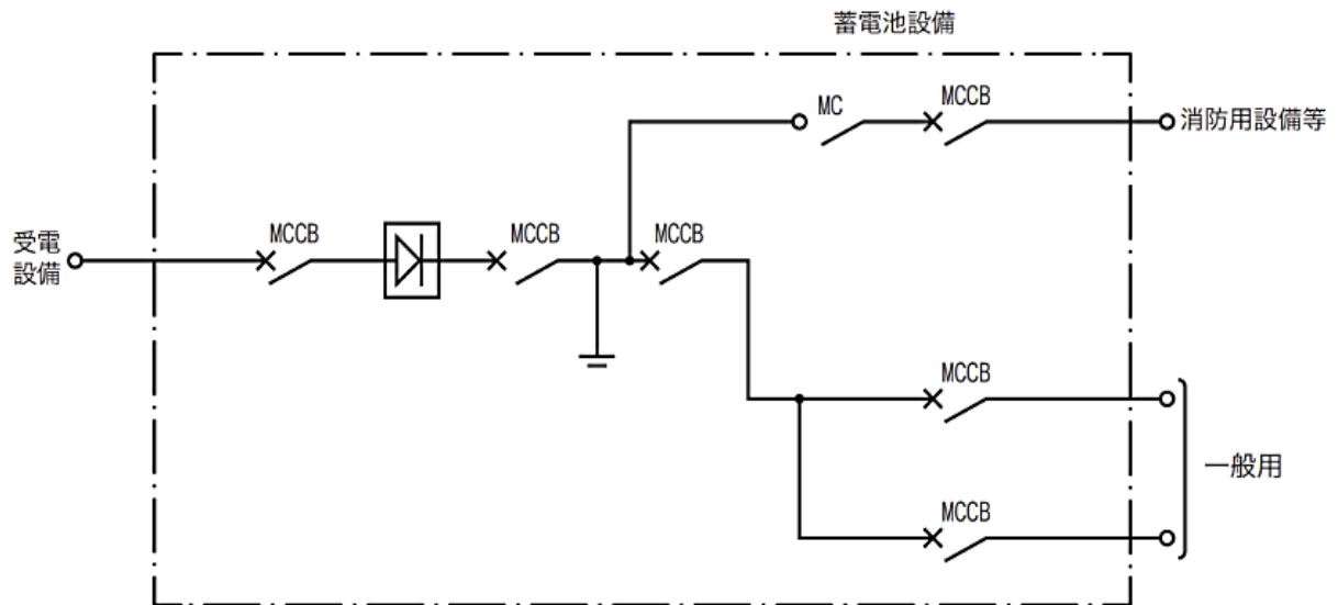
別図5 蓄電池設備の分岐方法
