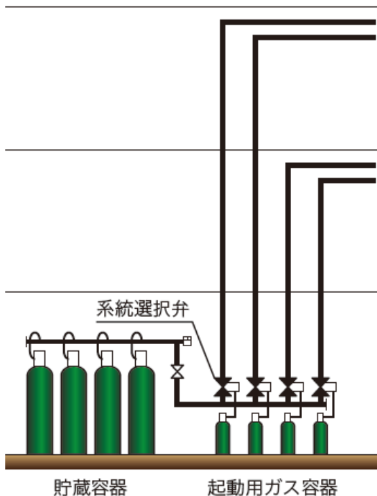
（一般的な配管方式の例）
