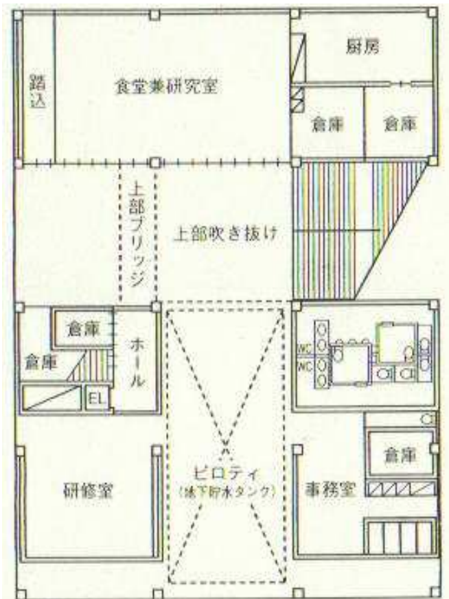
1 階平面図
