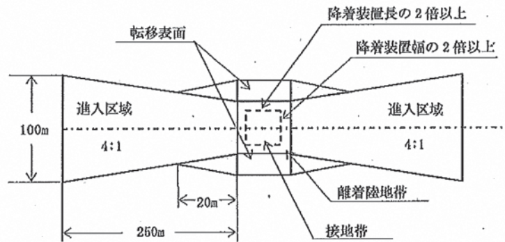
① 平面図
