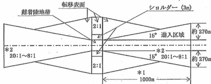
① 平面図
