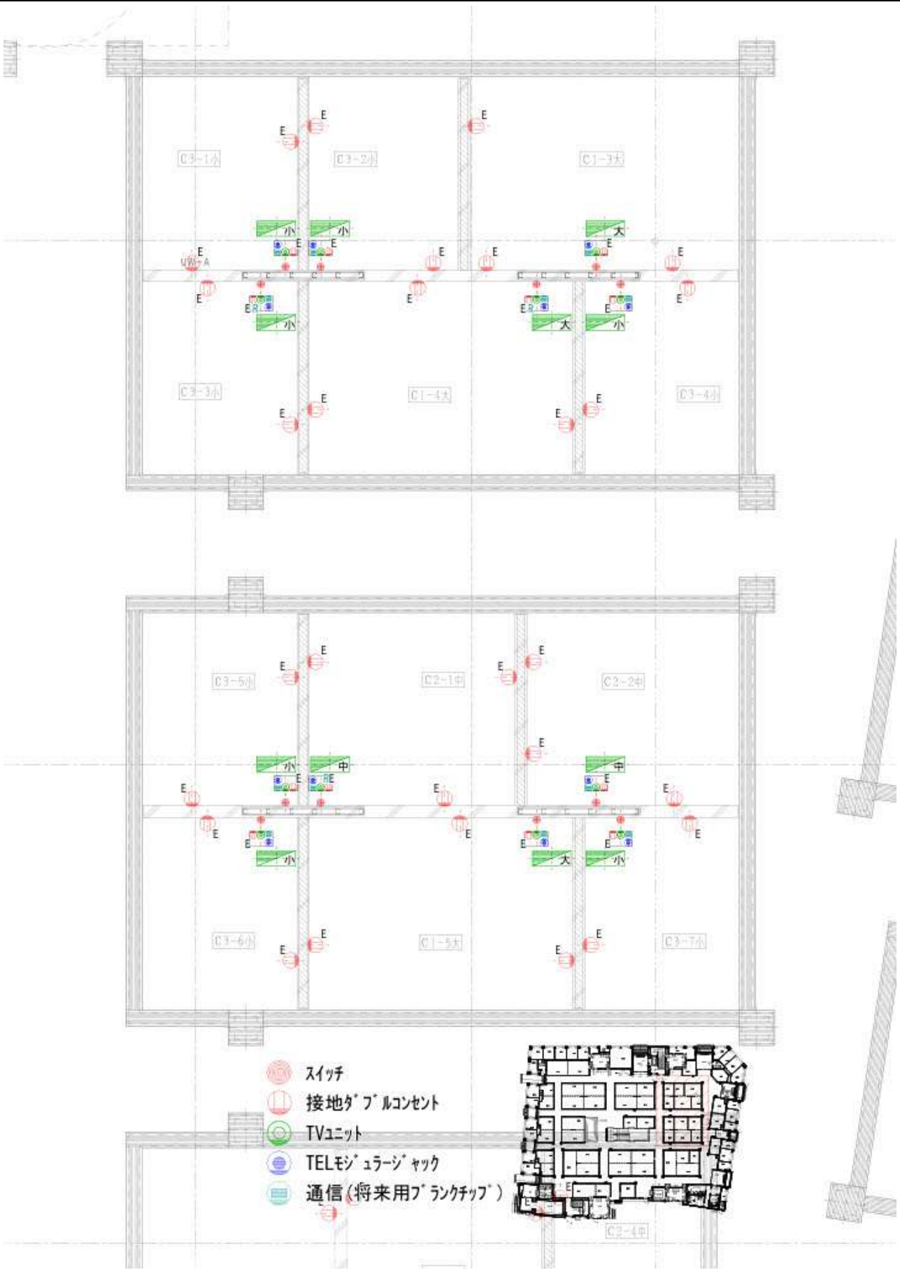
資料 電気平面図（生鮮部門一部エリア参考）
