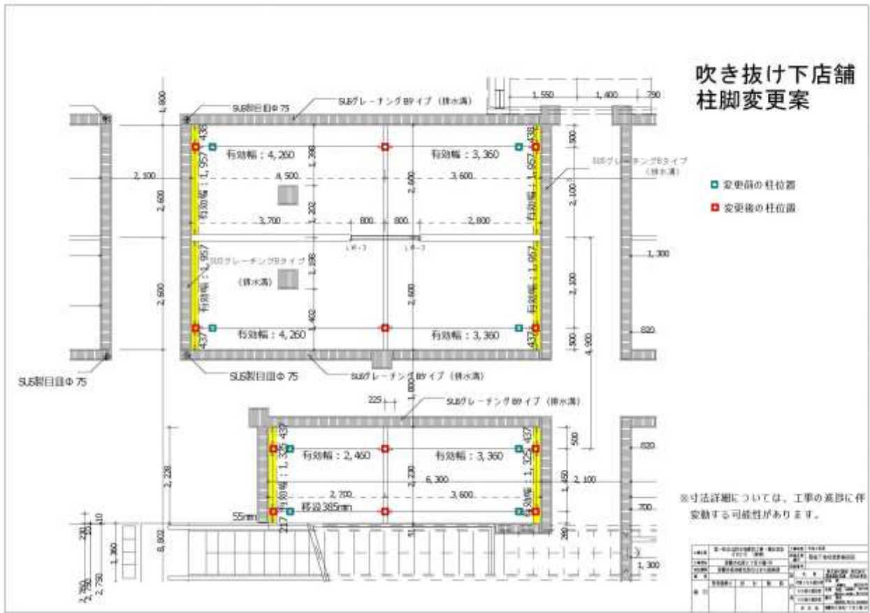
資料 吹き抜け下店舗柱脚変更案
