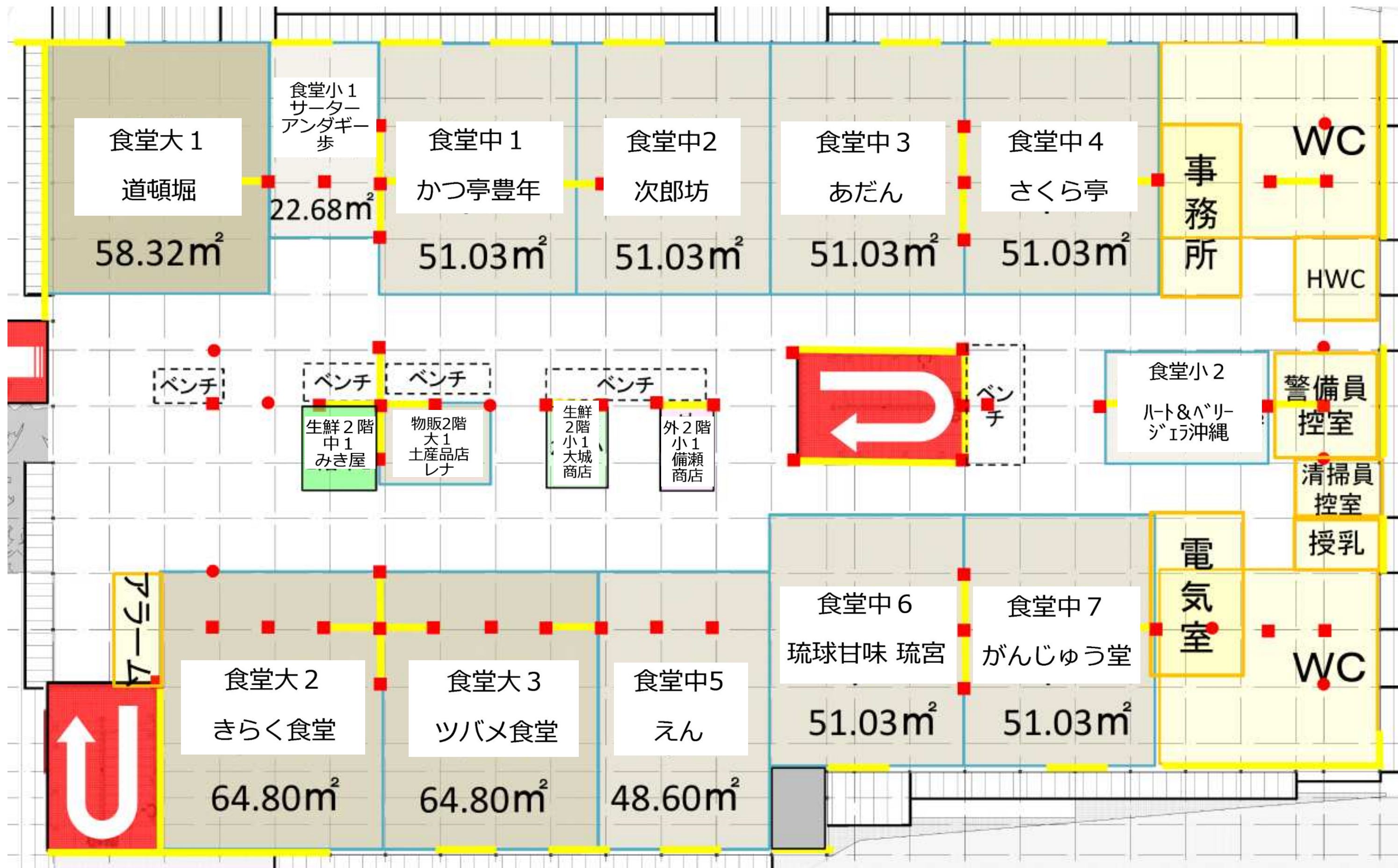
2 階平面図
