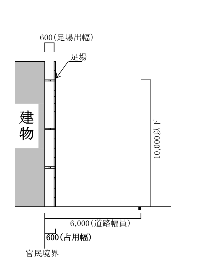
1道路幅員6,000 足場出幅600 足場高10,000以下
