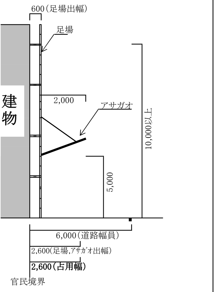
2道路幅員6,000 足場出幅600 足場高10,000以上
