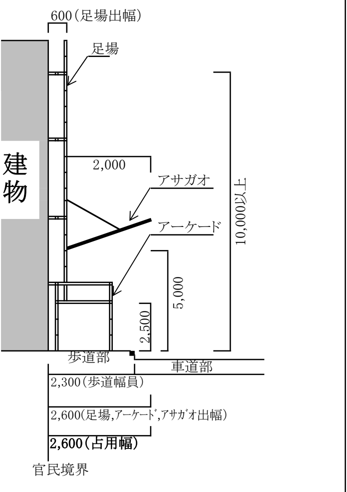
4歩道幅員2,300 足場出幅600 足場高10,000以上
