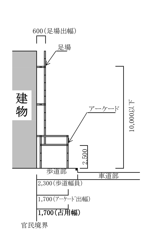
3歩道幅員2,300 足場出幅600 足場高10,000以下
