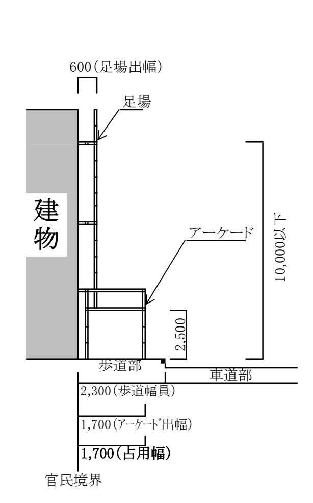
3歩道幅員2,300 足場出幅600 足場高10,000以下
