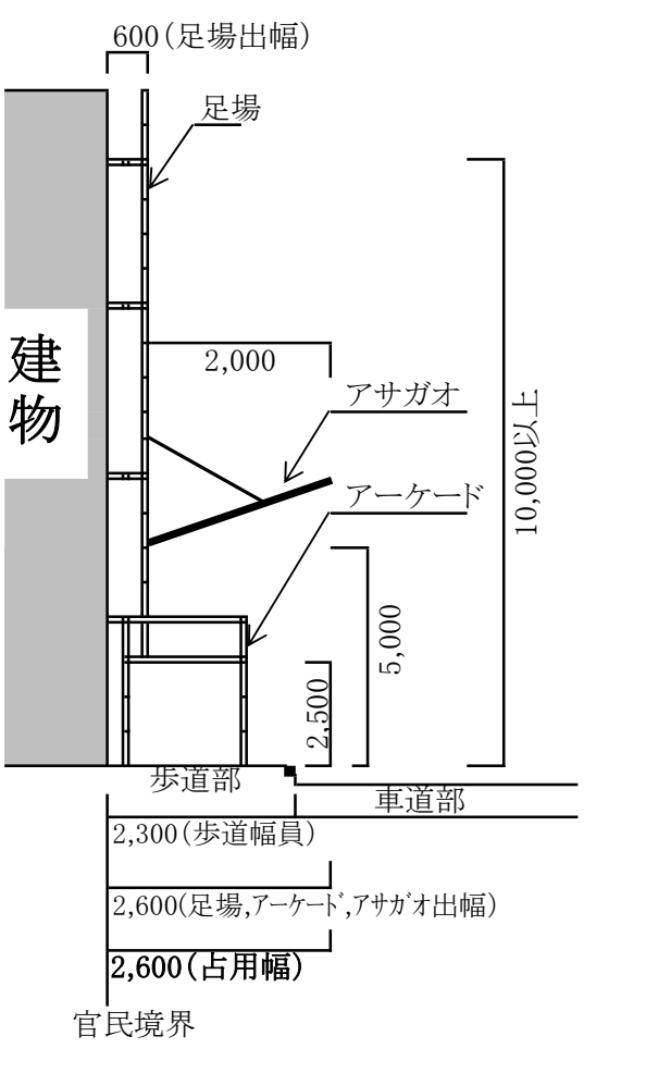
4歩道幅員2,300 足場出幅600 足場高10,000以上
