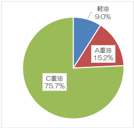
図4-2-15 船舶（旅客）の燃料種別排出量内訳（2022年度）
