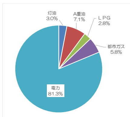
図4-2-21 民生業務部門の燃料種別排出量内訳（2022年度）
