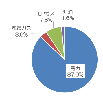
図4-2-17 民生家庭部門の燃料種別排出量内訳（2022年度）
