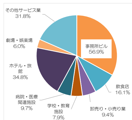
図4-2-22 業種別排出量内訳（2022年度）
