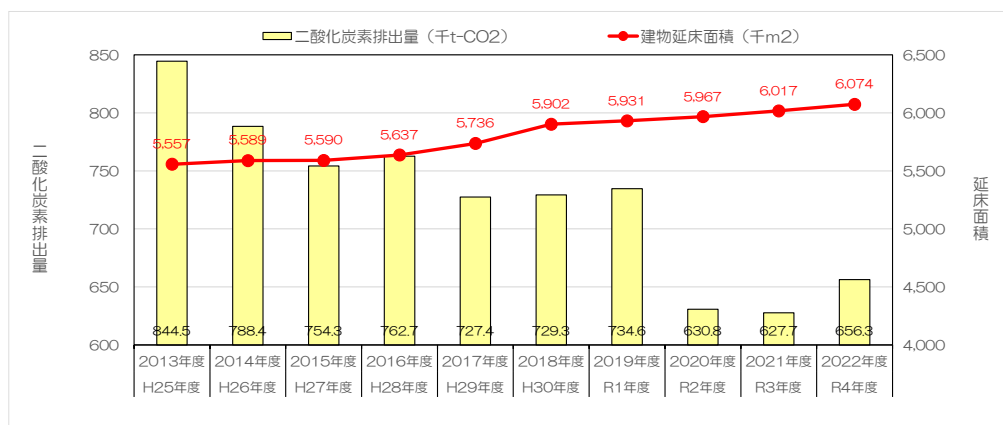
図4-2-23 民生業務部門における二酸化炭素排出量と建築延床面積
