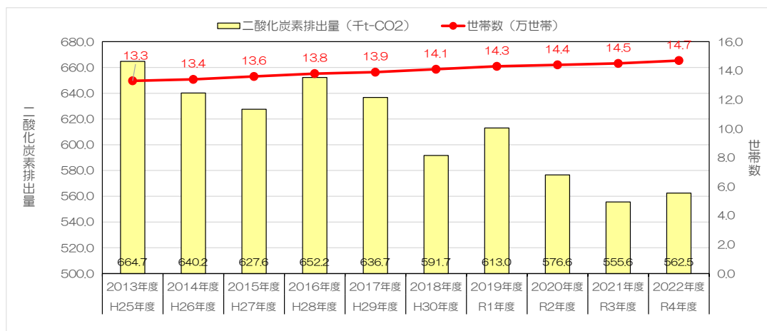
図4-2-18 民生家庭部門における二酸化炭素排出量と世帯数
