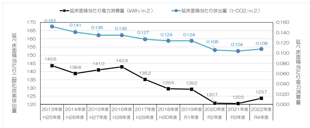
図4-2-26 民生業務部門における延床面積当たり二酸化炭素排出量及び電力消費量
