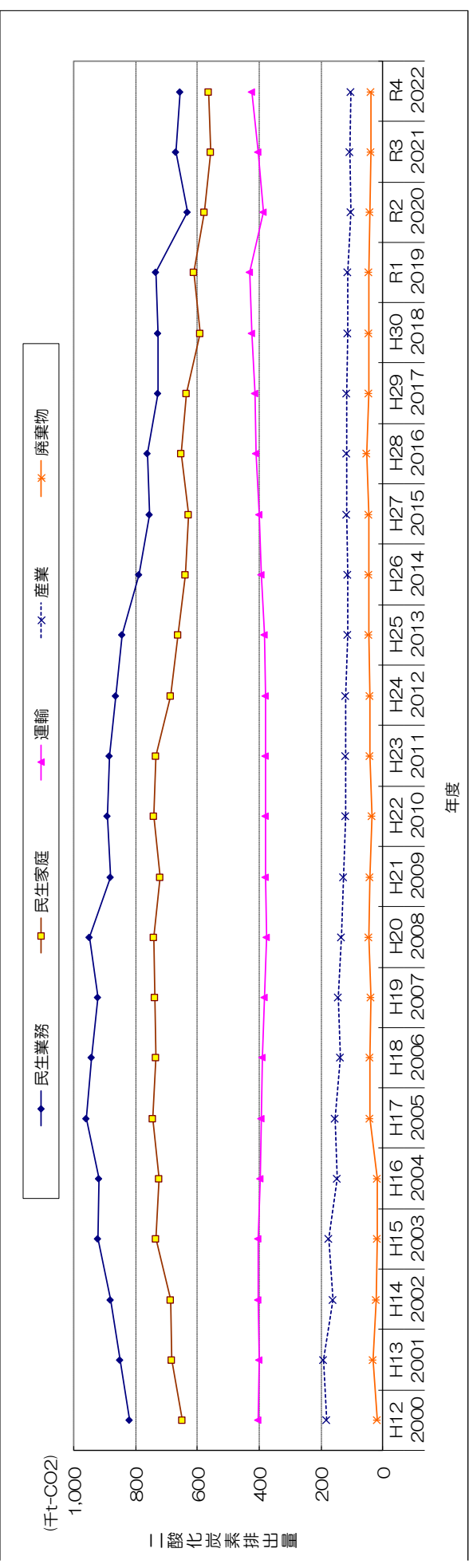
図-3-2 那覇市二酸化炭素排出量の推移（2000年度-2022年度）
