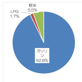
図4-2-8 自動車の燃料種別排出量内訳（2022年度）
