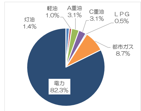
図4-2-1 製造業の燃料種別排出量内訳（2022年度）
