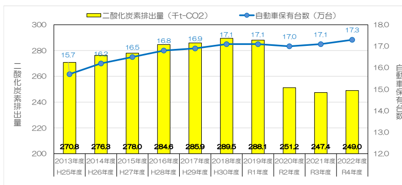
図4-2-9 自動車における二酸化炭素排出量と保有台数
