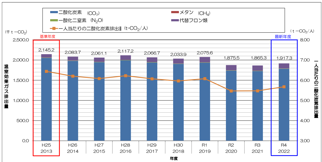
図3-1 那覇市における温室効果ガス排出量の推移
