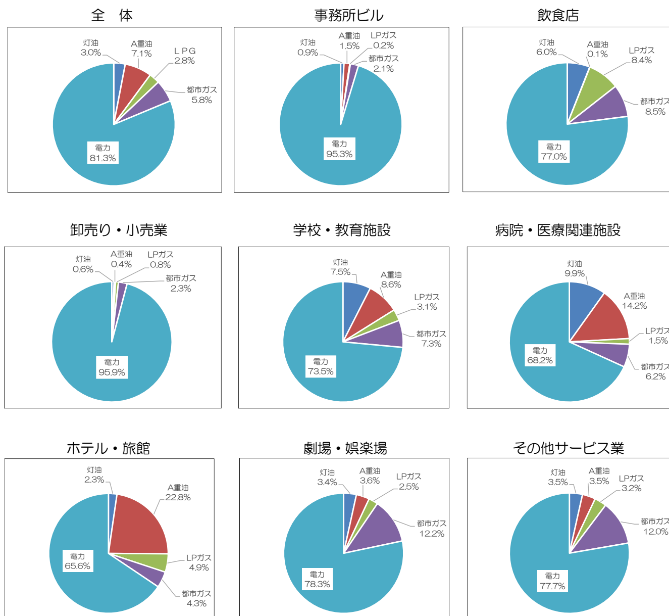
図 4-2-27 民生業務部門における業種別の燃料種別二酸化炭素排出量の内訳（2022 年度）
