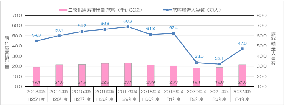
図4-2-13 船舶（旅客）における二酸化炭素排出量
