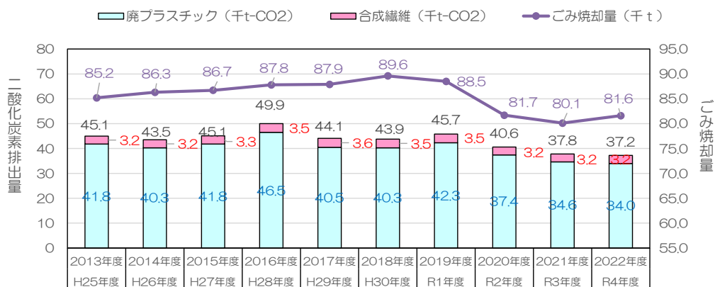
図4-2-29 一般廃棄物における二酸化炭素排出量及びごみ焼却量
