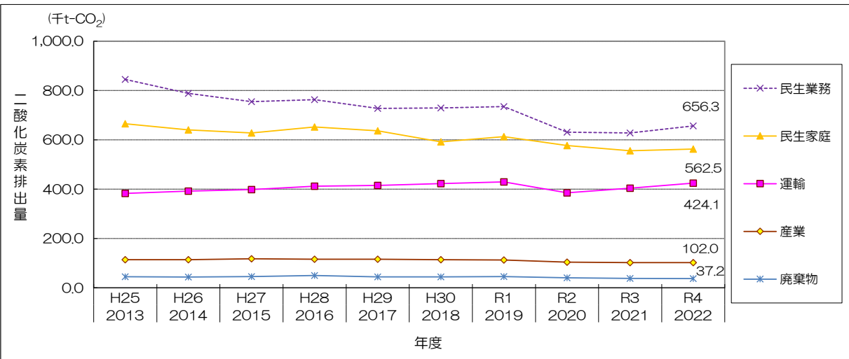
図4-1-1 那覇市の部門別二酸化炭素排出量の推移
