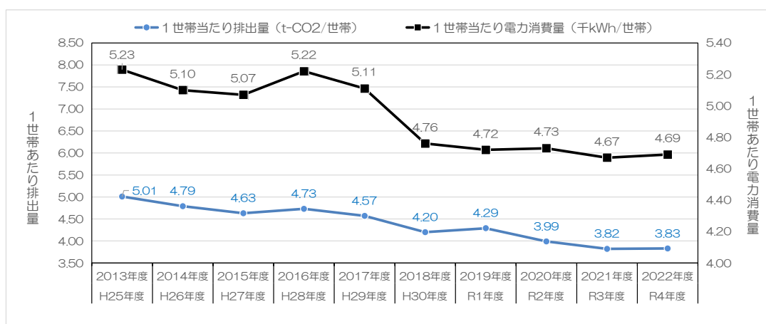
図4-2-20 民生家庭部門における1世帯当たりの二酸化炭素排出量・電力消費量
