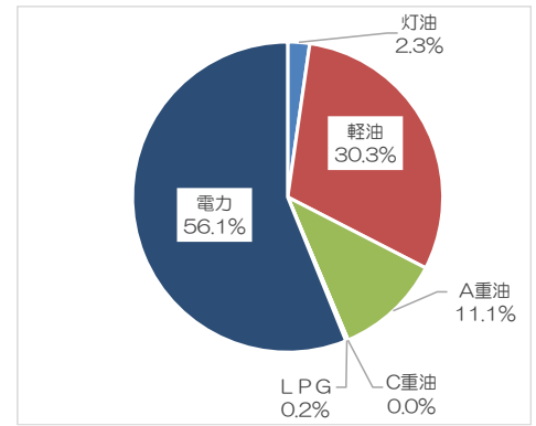
図4-2-5 鉱業建設業の燃料種別排出量内訳（2022年度）
