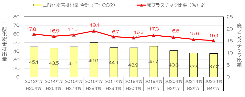
図4-2-30 一般廃棄物における二酸化炭素排出量及び廃プラスチックの比率
