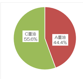
図4-2-16 船舶（貨物）の燃料種別排出量内訳（2022年度）
