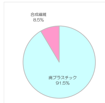
図4-2-28 一般廃棄物の種類別排出量内訳（2022年度）
