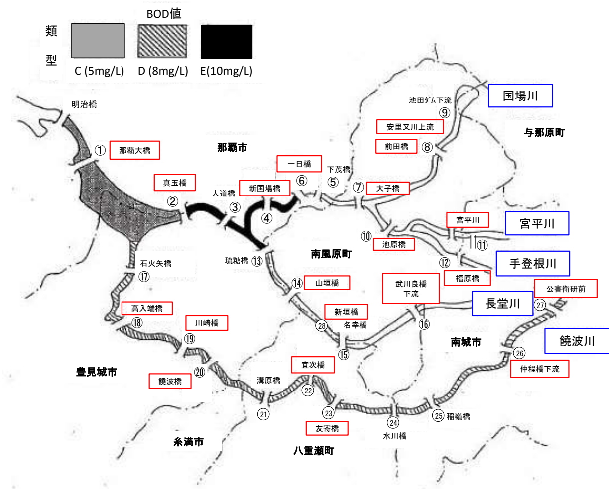
図 6 - 4 調査地点図
